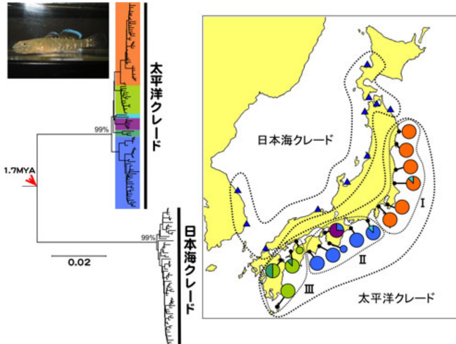
図1. 日本列島沿岸におけるアゴハゼ集団の遺伝的分化. アゴハゼは日本列島の潮間帯で普通に見られますが, そのミトコンドリアDNAの系統は太平洋側と日本海側とで大きく2つに分かれており, これらは170万年前に分岐したことが明らかにされました (Hirase et al. , 2012).
